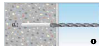
1 קידוחו חור
